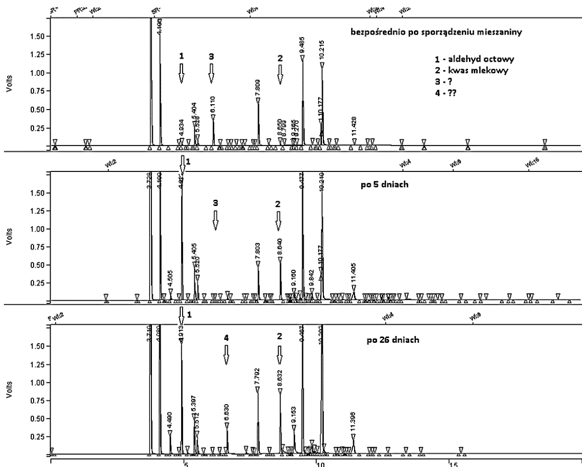
Rys. 2. Wpływ czasu od pobrania do analizy próbki mieszaniny wzorcowej (GC-FID). Fig. 2. Influence of time from sampling to analysis of mixture of model compounds (GC-FID).
